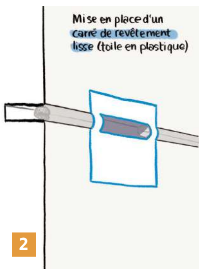
Étapes de pose d'un dispositif anti-retour pour les chauves-souris
